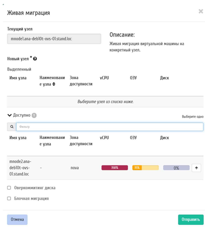
Рисунок 69 Окно запуска миграции виртуальной машины
