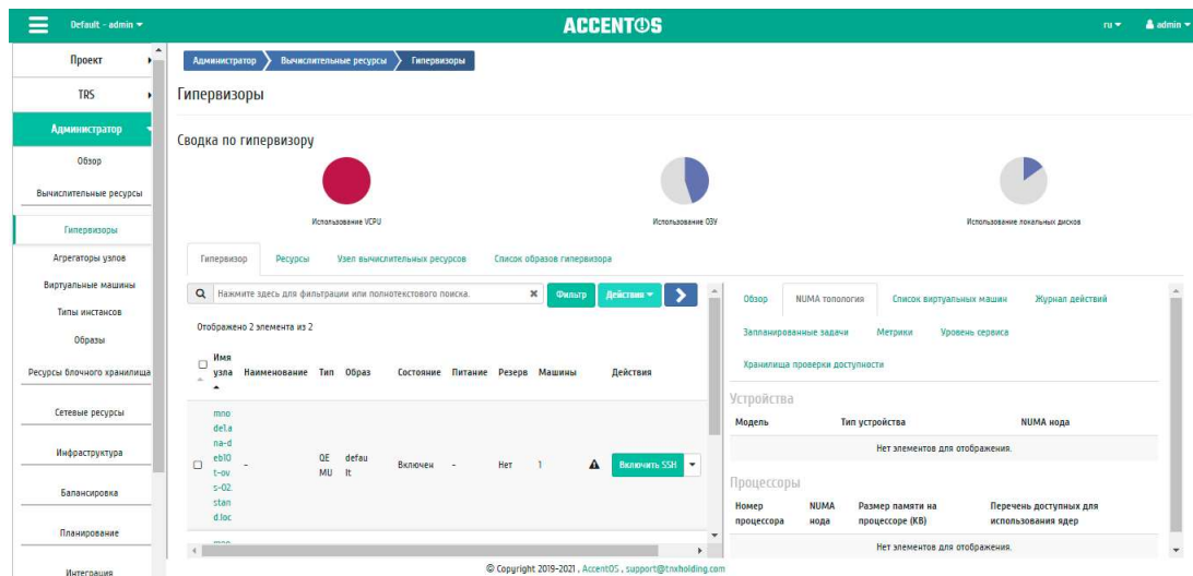
Рисунок 11 NUMA топология гипервизора
