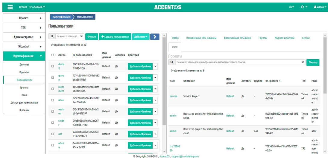
Рисунок 337 Список проектов и доменов пользователя
