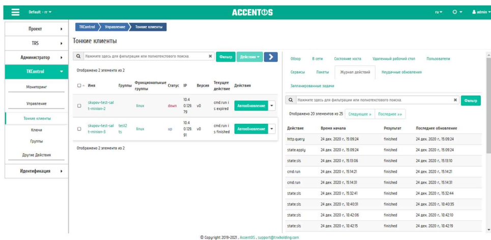
Рисунок 267 Журнал действий тонкого клиента
