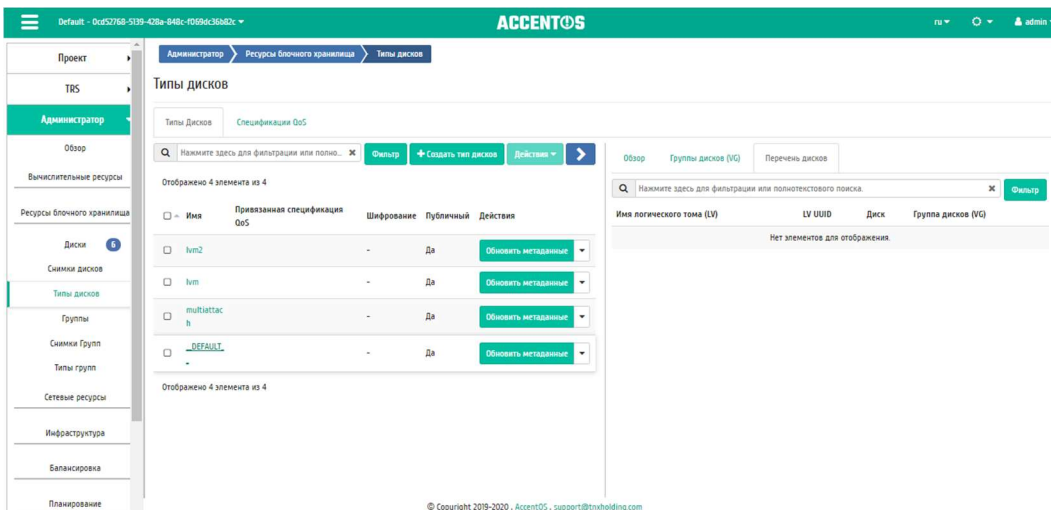
Рисунок 119 Перечень дисков
