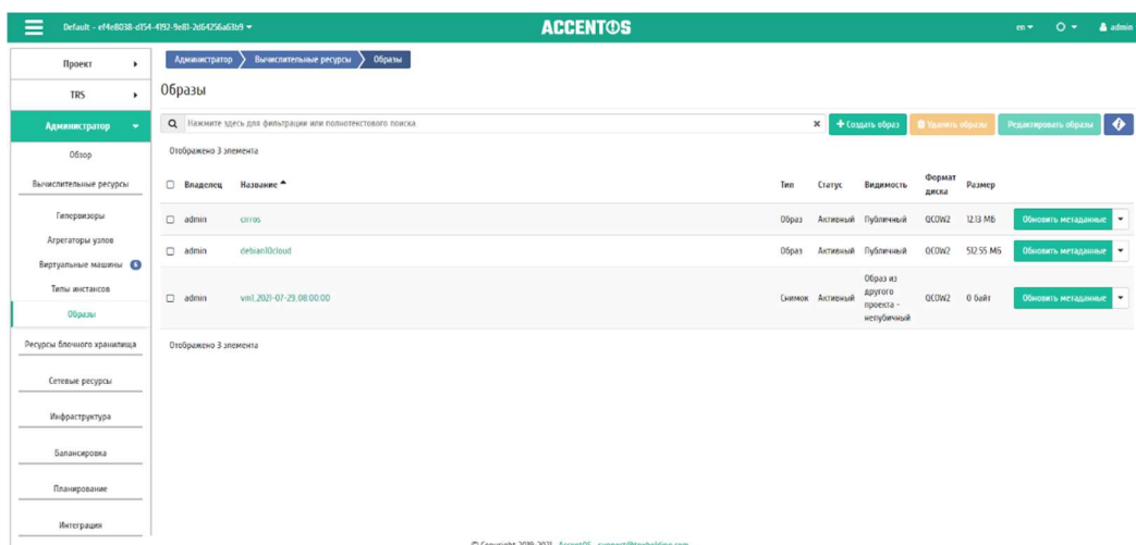
Рисунок 88 Список образов
