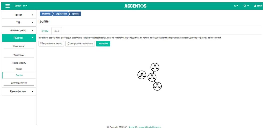
Рисунок 280 Граф
