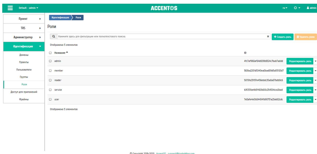
Рисунок 357 Список ролей
