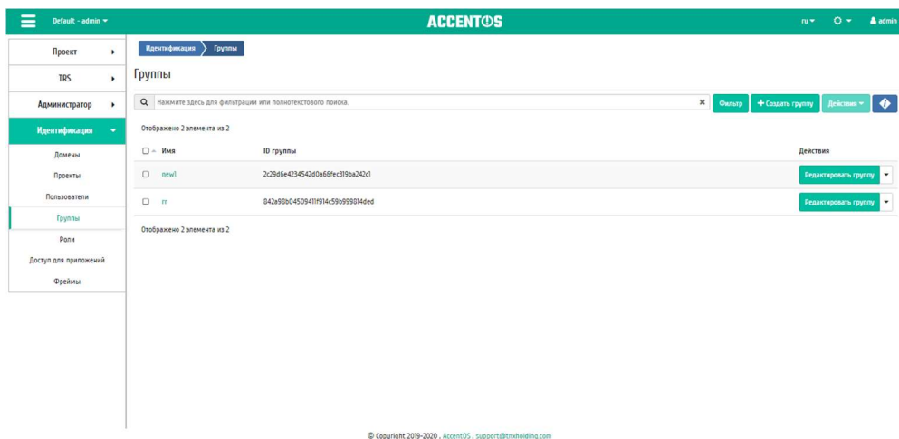
Рисунок 348 Список групп
