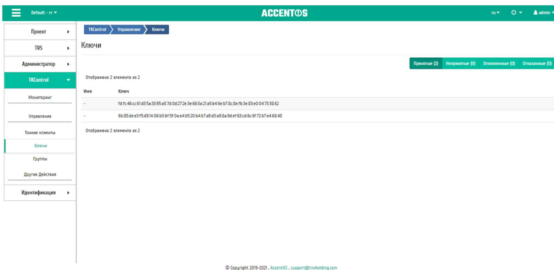
Рисунок 272 Список ключей
