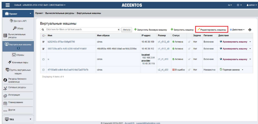
Рисунок 392 Групповое редактирование
