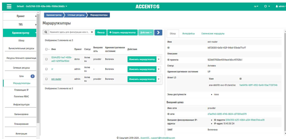
Рисунок 161 Подробные параметры маршрутизатора
