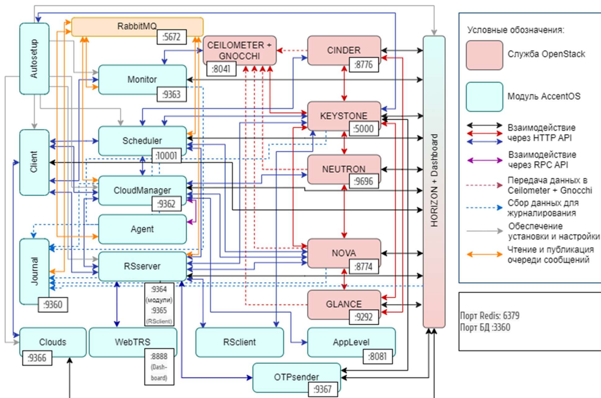
Рисунок 1 Архитектура решения
