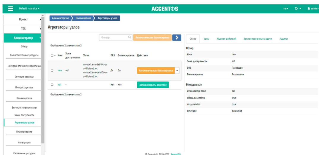
Рисунок 214 Подробные параметры агрегатора узлов
